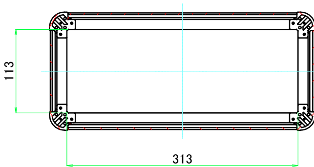
C-C ( 1 : 5 )
