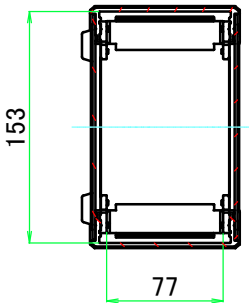
A-A ( 1 : 5 )
